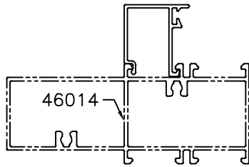
46014 SCALE :-1:2
