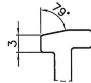
DETAIL-A SCALE 2:1
