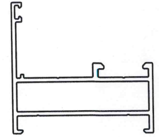
SCALE 1:1
