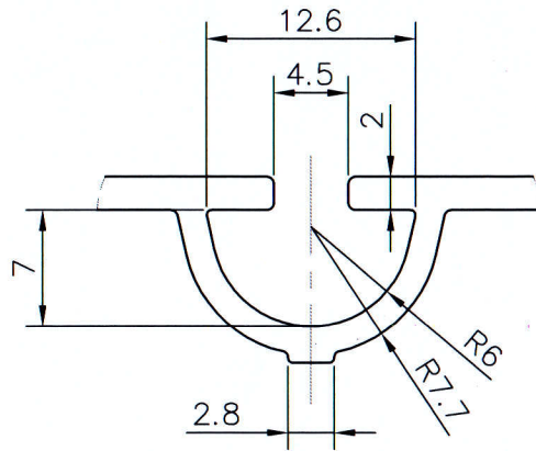
DETAIL-A SCALE 2:1
