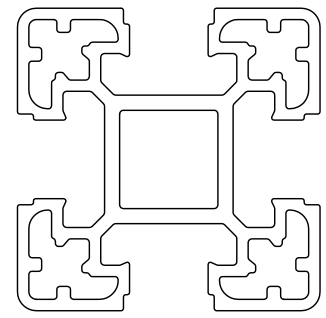
SCALE 1:1
