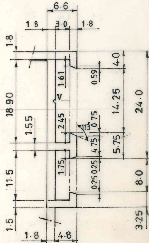
DETAIL-B
