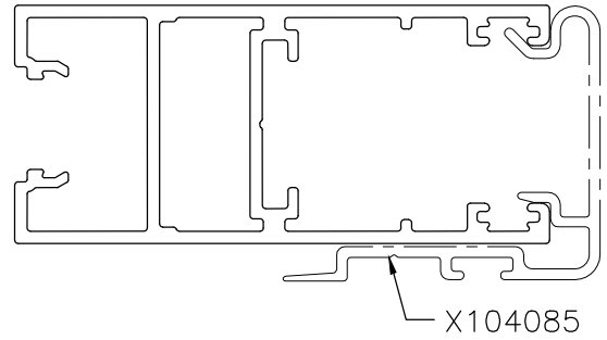
MATCHING SCALE 1:1
