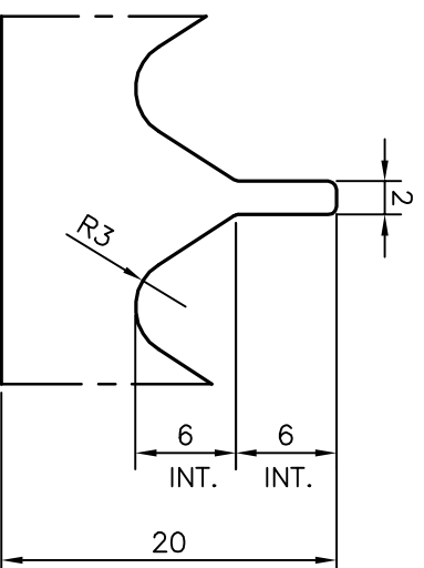
DETAIL 'A' SCALE 2:1
