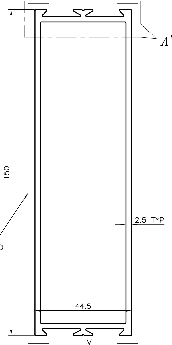
DETAIL-A SCALE: -2:1
