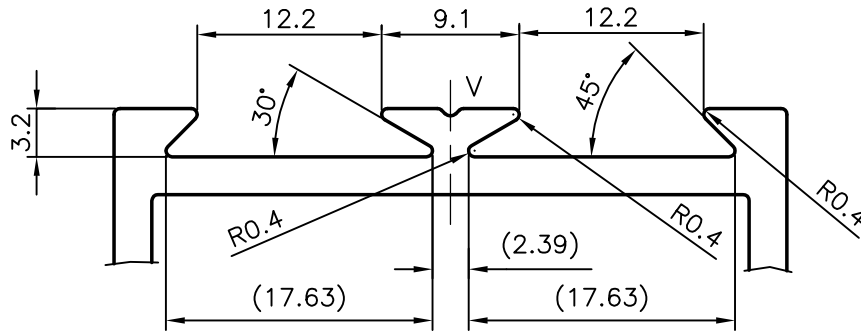
DETAIL-A SCALE: -2:1
