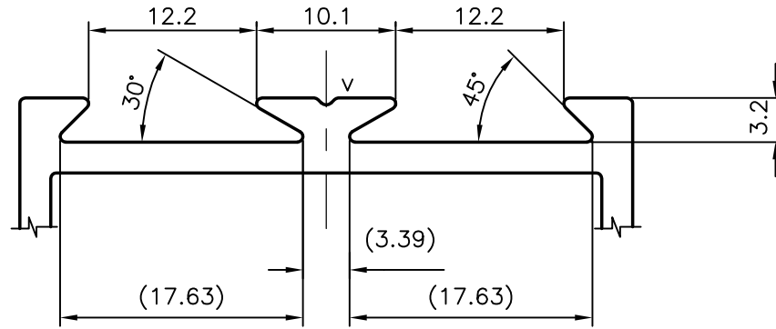
DETAIL-A SCALE: -2:1
