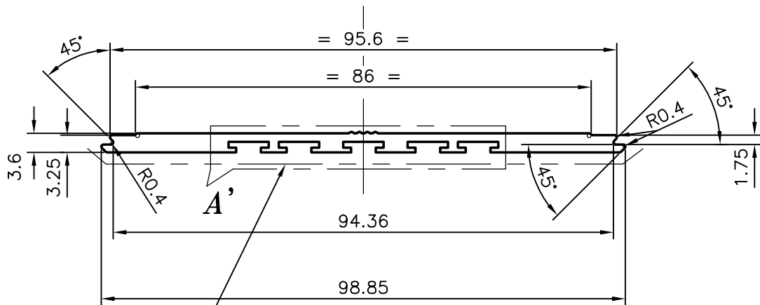
DETAIL-A SCALE:2:1
