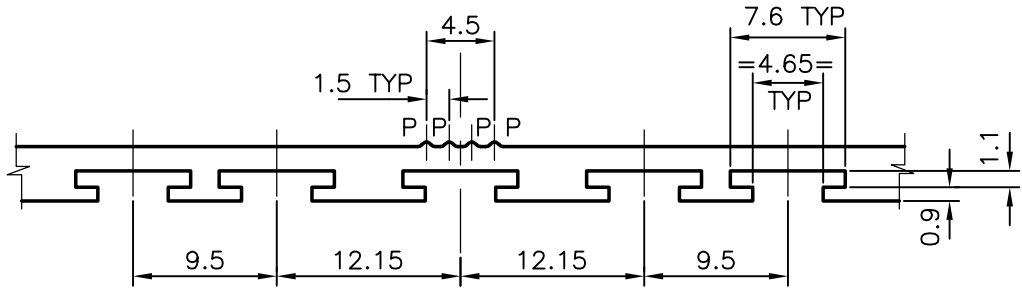
DETAIL-A SCALE:2:1
