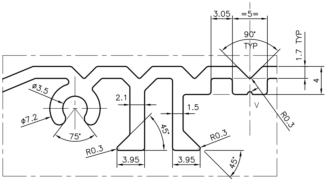
DETAIL-A SCALE: -3:1
